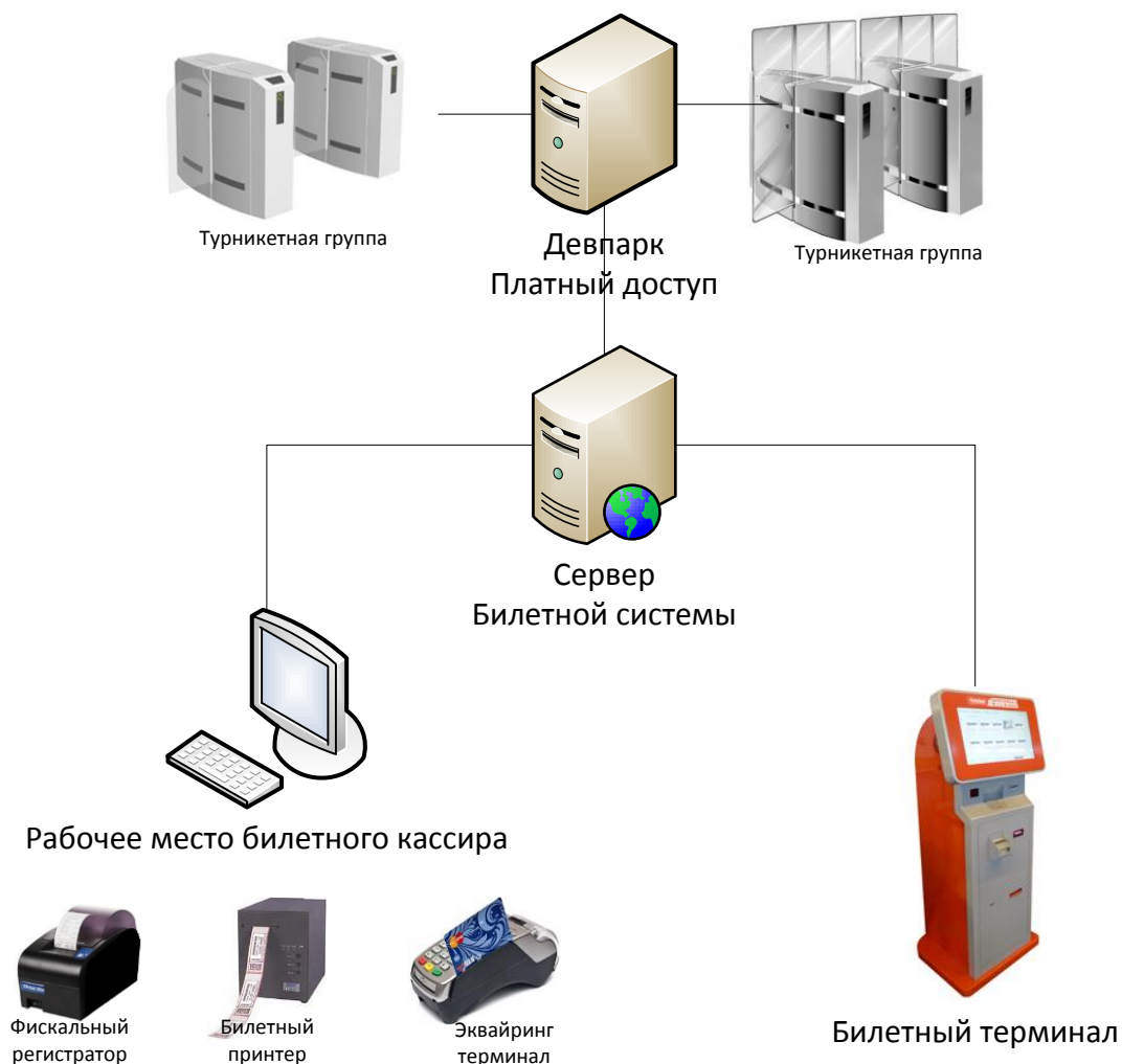
Схема компонентов билетной системы
